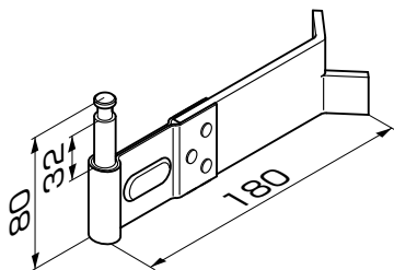
図1-2 AUS、AUW姿図
