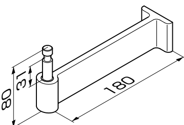
図1-3 VUS、VUW姿図
