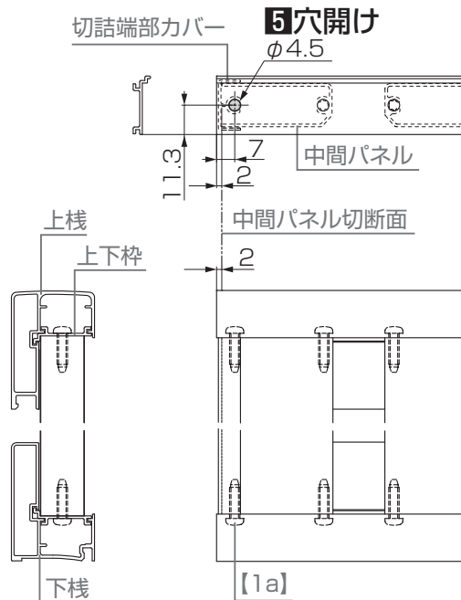
【図2-3 上下枠の加工】
