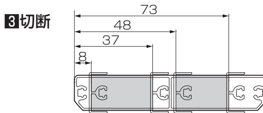
【図2-2 中間パネル縦割り可能範囲】
