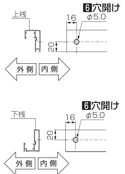
【図2-4 上棧・下棧の加工】
