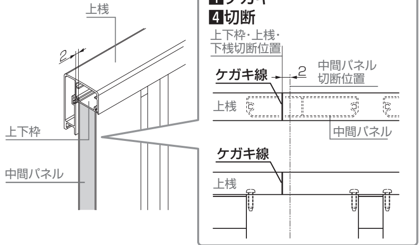
【図2-1 上下枠・上棧・下棧の切断位置】
