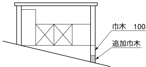
図1-1 傾斜地での取付け位置
