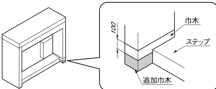
図1-3 ステップ施工時での取付け位置
