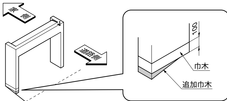
図1-2 水勾配地での取付け位置
