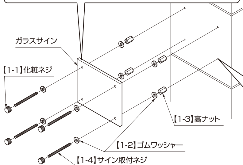
図1-2 サイン組み立て(ベーシックタイプ)
