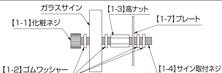
図1-3 サイン組み立て(プレート付きタイプ)
